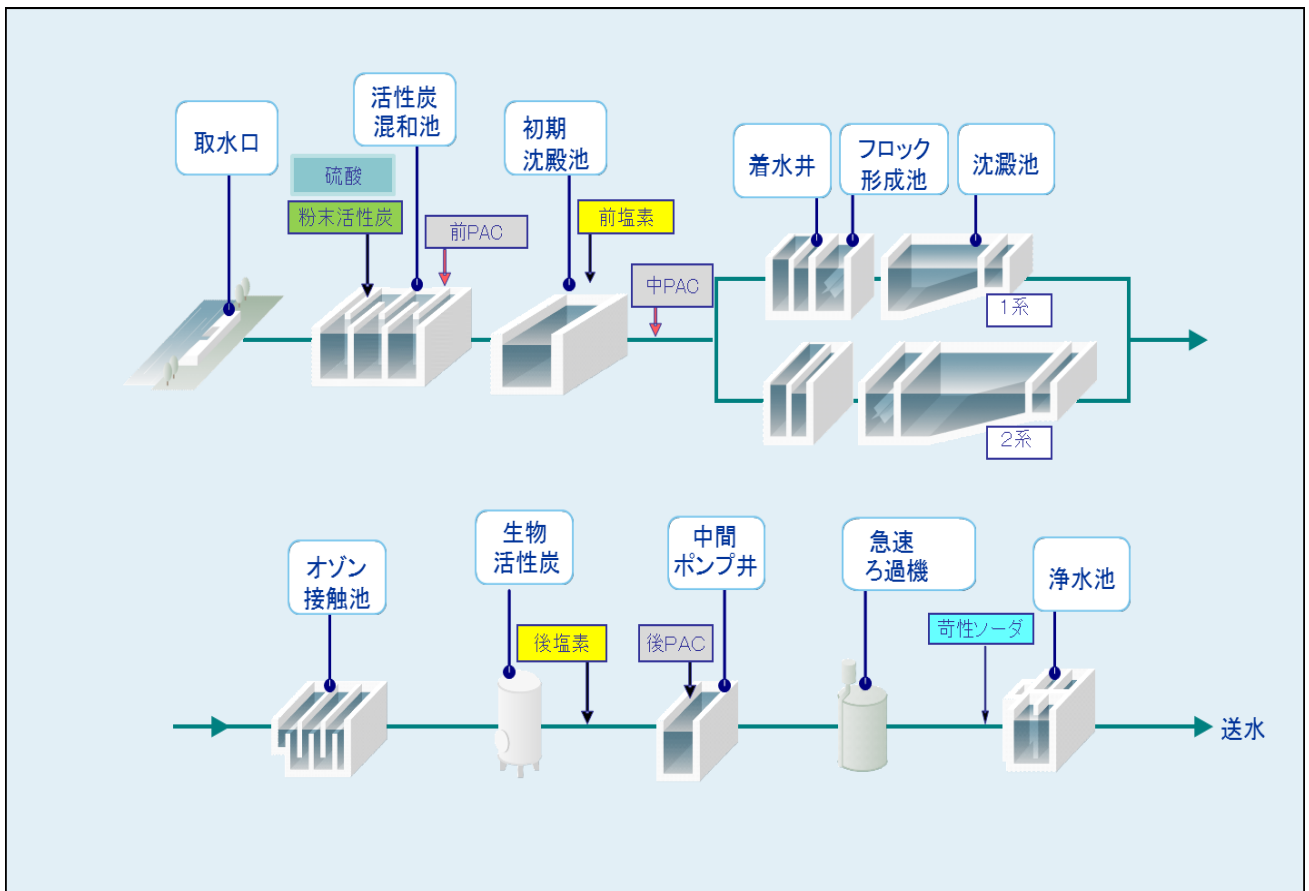
【図-2】前新田浄水場 浄水処理フロー
